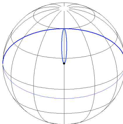
Abbildung 1: Bahnebene und Keplerellipse
